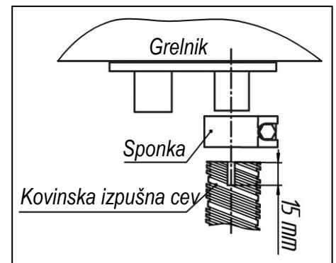
Slika 8 - Pritrditev kovinske cevi na grelnik
