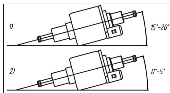
Slika 18 - Način namestitve črpalke za gorivo Advers (1) in črpalke za gorivo Thomas Magnete (2).
