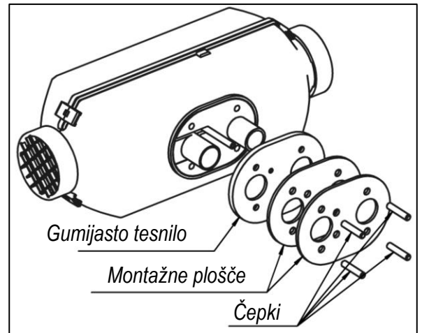
Slika 2a - Montažne plošče
